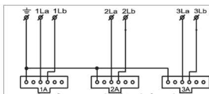
Schéma zapojení trojzásuvky
