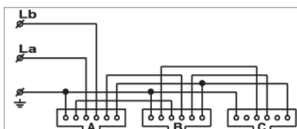
Schéma zapojení trojzásuvky (priorita A, B, C) TZ - ABCb 4 FK 282 21, 22, 45, 46, 81, 91.1
