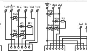
Schéma zapojení trojzásuvky průběžné TZÚP - 1A/2A2Bb 4 FK 282 61, 62, 84, 94.4
