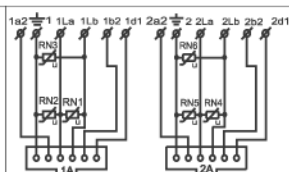
Schéma zapojení dvojzásuvky průběžné TZP - 1A/2Ab 4 FK 282 59, 60, 83, 93.3
