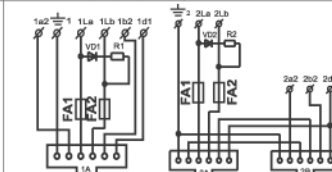
Schéma zapojení trojzásuvky průběžné TZÚP - 1A/2A2Bbn 4 FK 282 61.5, 61.5/F, 62.5, 94.5
