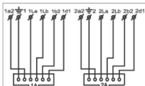
Schéma zapojení dvojzásuvky průběžné TZP - 1A/2Ab 4 FK 282 59, 60, 83, 93.1
