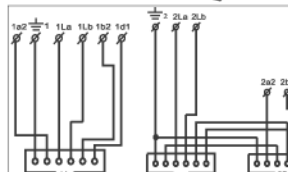
Schéma zapojení trojzásuvky průběžné TZP - 1A/2A2Bb 4 FK 282 61, 62, 84, 94.1
