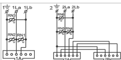
Schéma zapojení trojzásuvky TZ - 1A/2A2Bb 4 FK 282 35, 36, 41, 42, 80, 90.3
