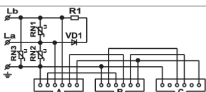
Schéma zapojení trojzásuvky (priorita A, B, C) TZÚ - ABCb 4 FK 282 21, 22, 45, 46, 81, 91.4
