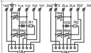
Schéma zapojení dvojzásuvky průběžné TZÚP - 1A/2Ab 4 FK 282 59, 60, 83, 93.4
