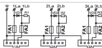
Schéma zapojení trojzásuvky
