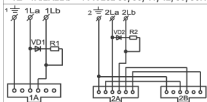
Schéma zapojení trojzásuvky TZÚ - 1A/2A2Bb 4 FK 282 35, 36, 41, 42, 80, 90.2
