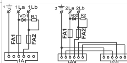
Schéma zapojení trojzásuvky TZÚ - 1A/2A2Bbn 4 FK 282 35.5, 35.5/F, 36, 80.5
