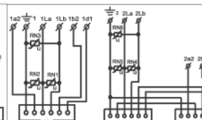
Schéma zapojení trojzásuvky průběžné TZP - 1A/2A2Bb 4 FK 282 61, 62, 84, 94.3
