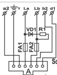
Schéma zapojení jednoduché zásuvky průběžné TZÚP - Ab 4 FK 282 57, 58, 69, 70, 82, 92.4
