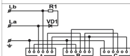
Schéma zapojení trojzásuvky (priorita A, B, C) TZÚ - ABCb 4 FK 282 21, 22, 45, 46, 81, 91.2
