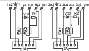
Schéma zapojení dvojzásuvky průběžné TZÚP - 1A/2Abn 4 FK 282 59.5, 59.5/F, 60.5, 83.5
