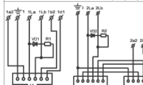
Schéma zapojení trojzásuvky průběžné TZÚP - 1A/2A2Bb 4 FK 282 61, 62, 84, 94.2
