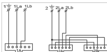
Schéma zapojení trojzásuvky TZ - 1A/2A2Bb 4 FK 282 35, 36, 41, 42, 80, 90.1
