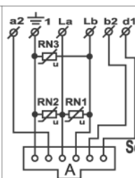
Schéma zapojení jednoduché zásuvky průběžné TZP - Ab 4 FK 282 57, 58, 69, 70, 82, 92.1
