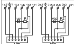
Schéma zapojení dvojzásuvky průběžné TZÚP - 1A/2Ab 4 FK 282 59, 60, 83, 93.2
