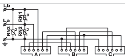
Schéma zapojení trojzásuvky (priorita A, B, C) TZ - ABCb 4 FK 282 21, 22, 45, 46, 81, 91.2
