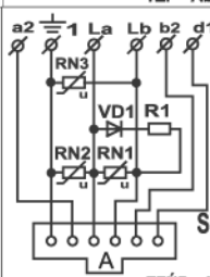
Schéma zapojení jednoduché zásuvky průběžné TZP - Ab 4 FK 282 57, 58, 69, 70, 82, 92.3
