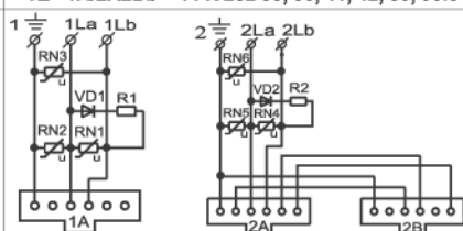
Schéma zapojení trojzásuvky TZÚ - 1A/2A2Bb 4 FK 282 35, 36, 41, 42, 80, 90.4
