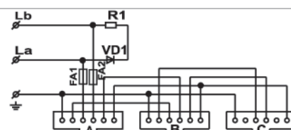
Schéma zapojení trojzásuvky (priorita A, B, C) TZÚ - ABCbn 4 FK 282 21, 22, 91.5
